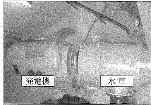
水車発電機 (イメージ)
