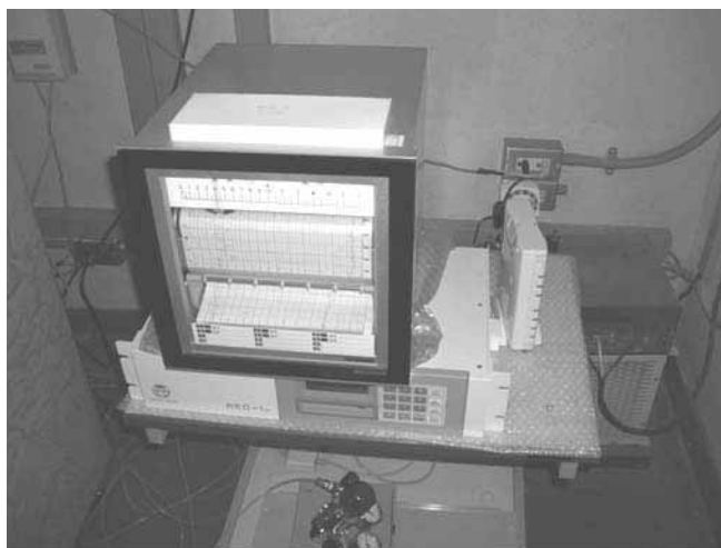
風向風速記録計(上) テレメータ装置(下)
