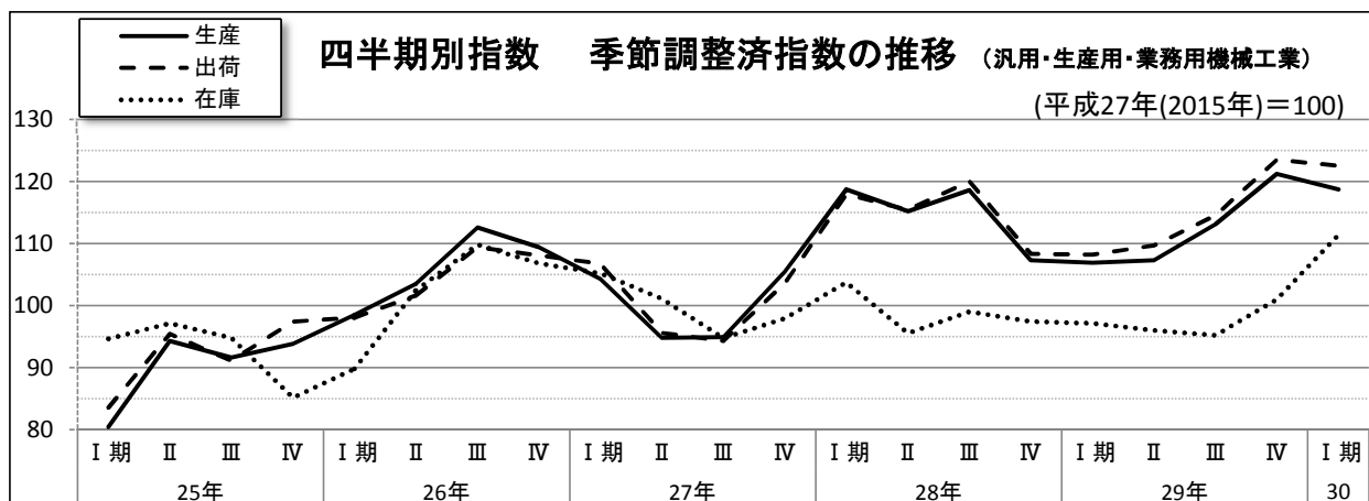
汎用・生産用・業務用機械工業 年別・四半期別指数の推移 (平成27年(2015年)=100)
