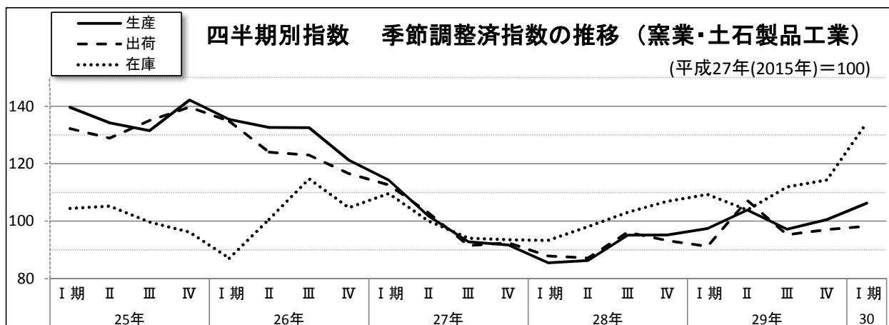
窯業・土石製品工業 年別・四半期別指数の推移 (平成27年(2015年)=100)
