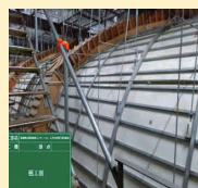
吊りボルト増設・ワイヤー増強
