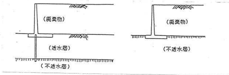
別図第1 コンクリート擁壁が遮水壁を兼ねる場合
