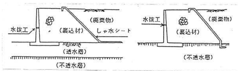
別図第2 コンクリート擁壁が遮水壁を兼ねない場合
