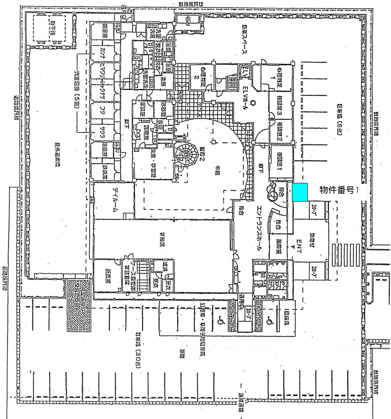
宮崎県北部福祉こどもセンター 配置図・1階平面図
