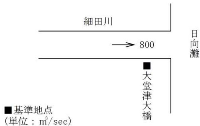
細田川計画高水流量図
