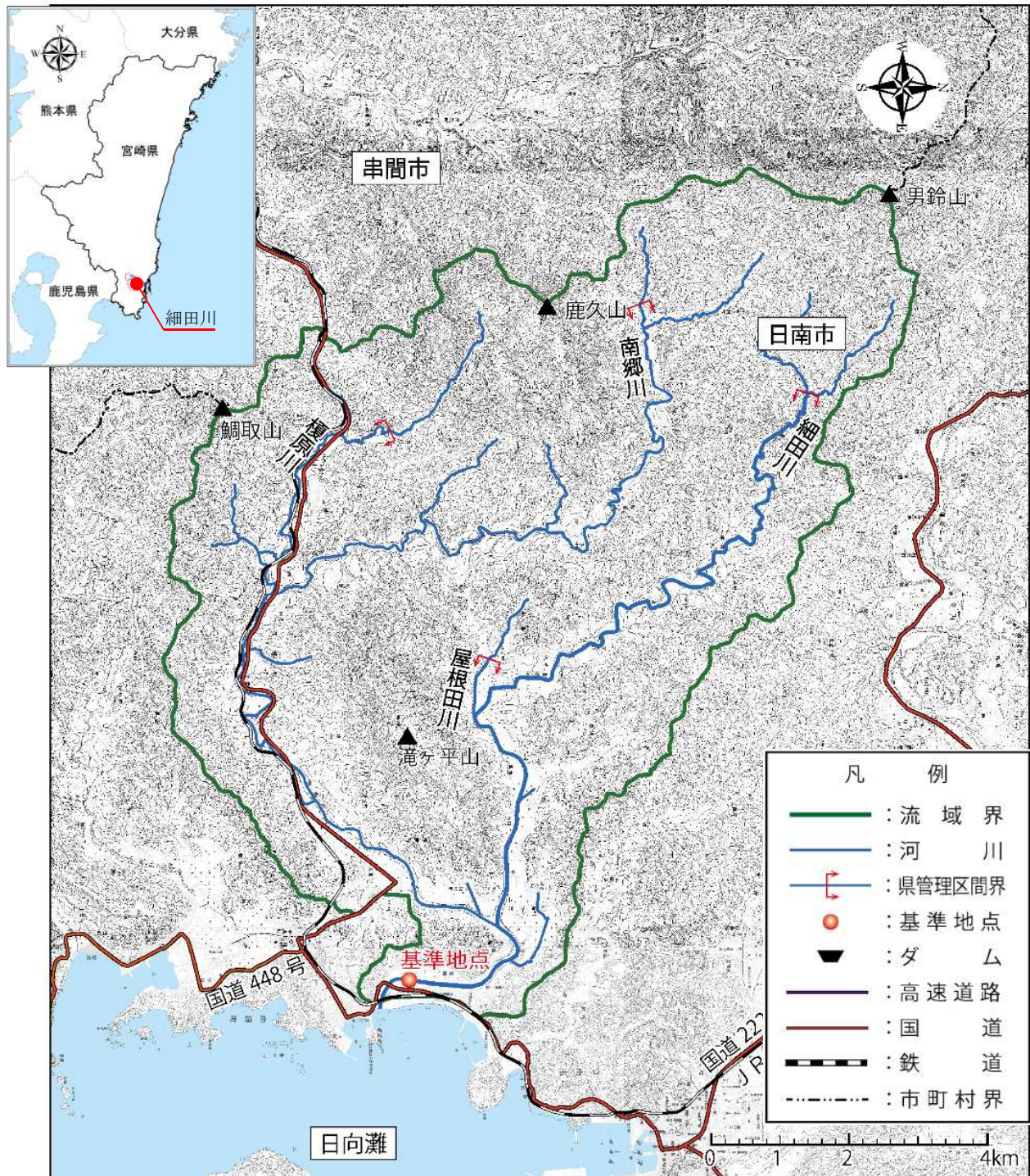
(参考図) 細田川水系図
