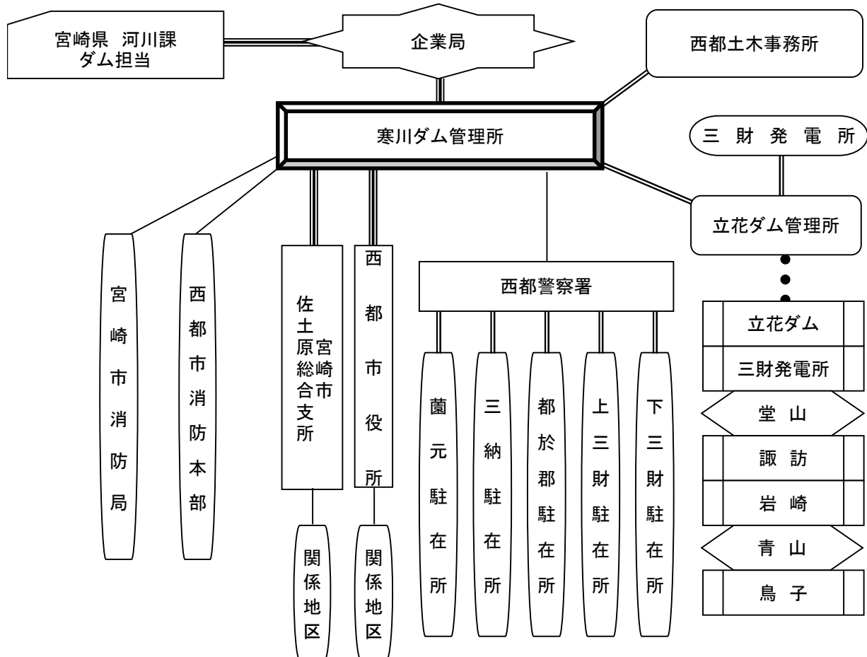
③②一ツ瀬川水系三財川 寒川ダム放流連絡系統図
