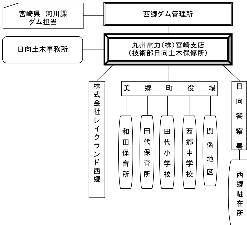
③0耳川水系耳川 西郷ダム放流連絡系統図
