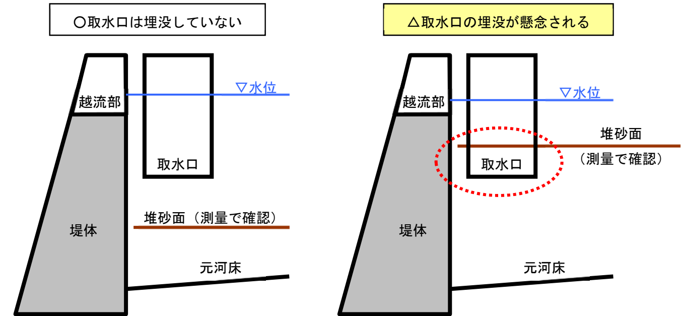
図11-1 堆砂形状と取水口高さの比較による取水口埋没評価イメージ
