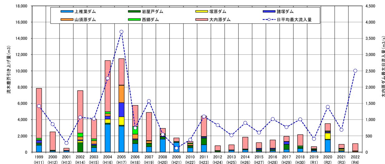
図12-1 流木塵芥引き上げ量と最大の推移
