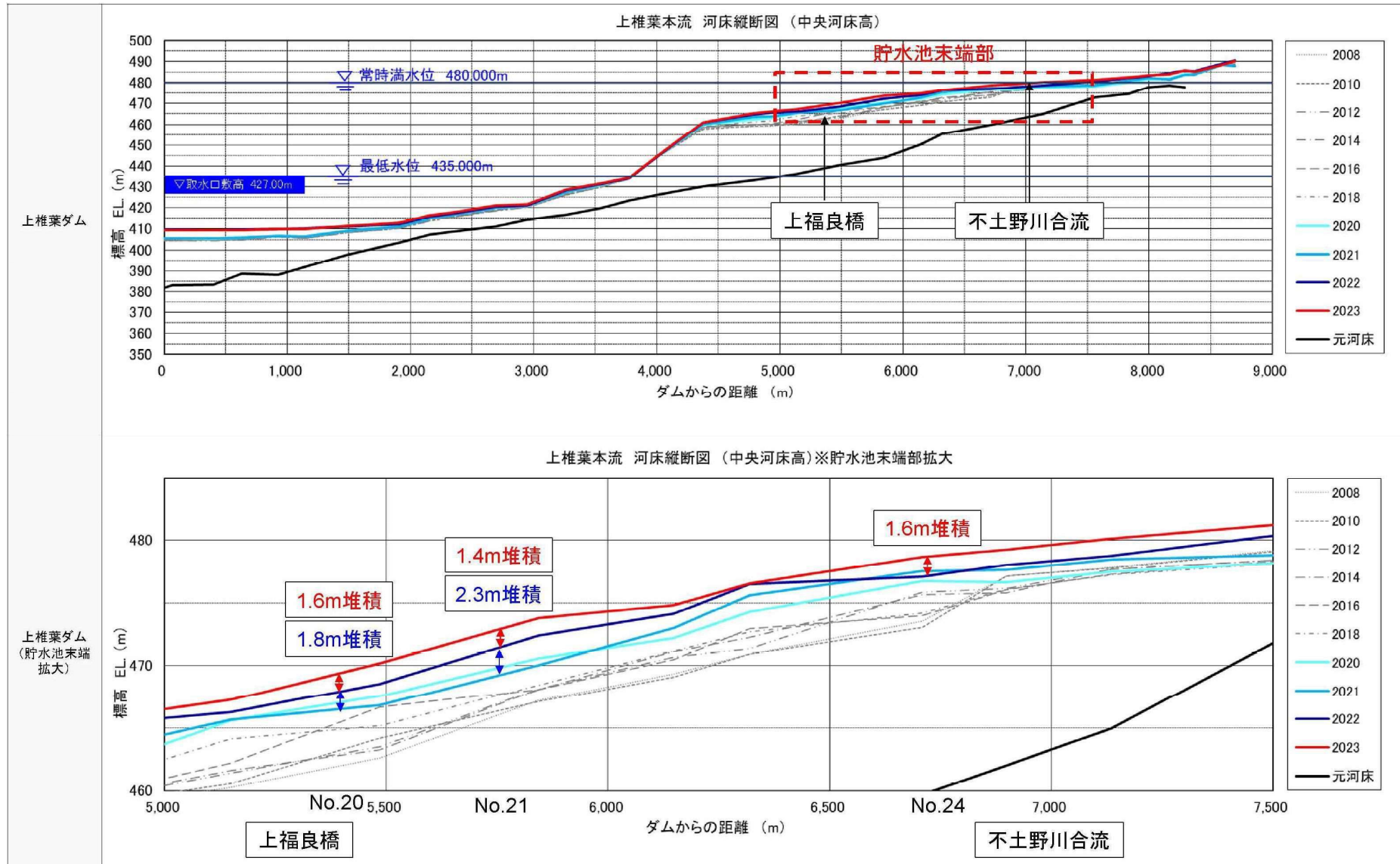
上椎葉ダム貯水池の河床縦断面図
