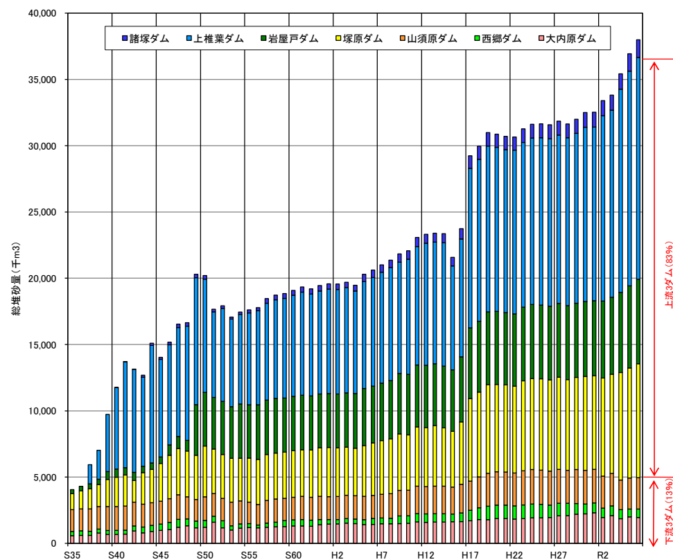
図1-6 ダム堆砂量の経年変化
