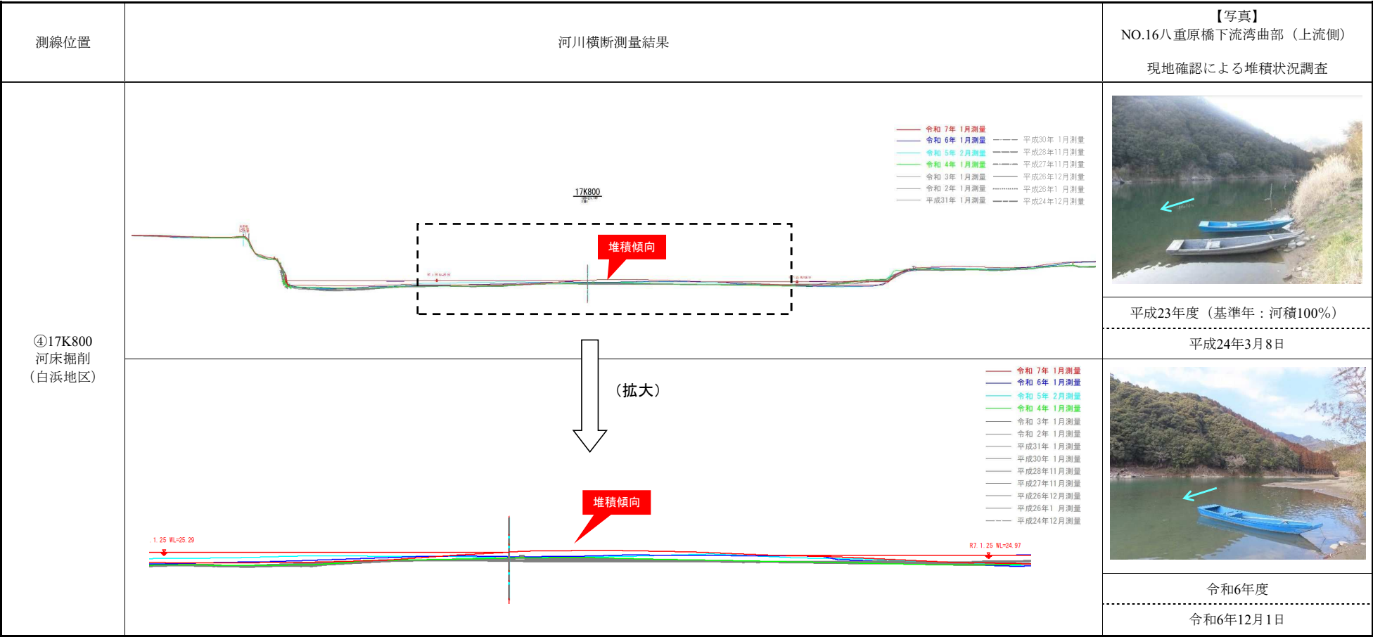
図 1-11 (3) 横断測量結果（治水安全度の評価対象箇所）
