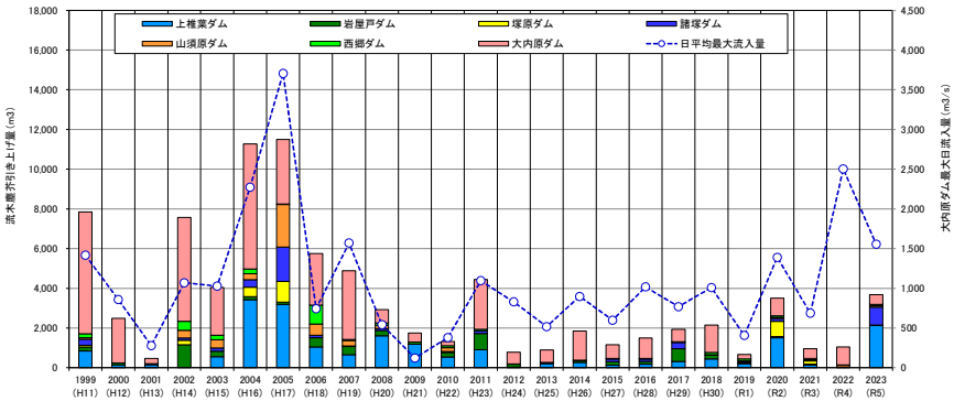
図5-4 流木塵芥引き上げ量と最大日流入量の推移
