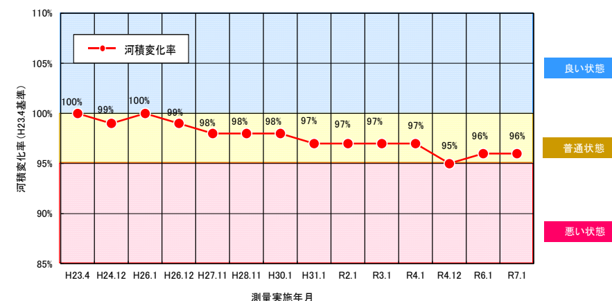
図1-10 河積変化率の経年変化
