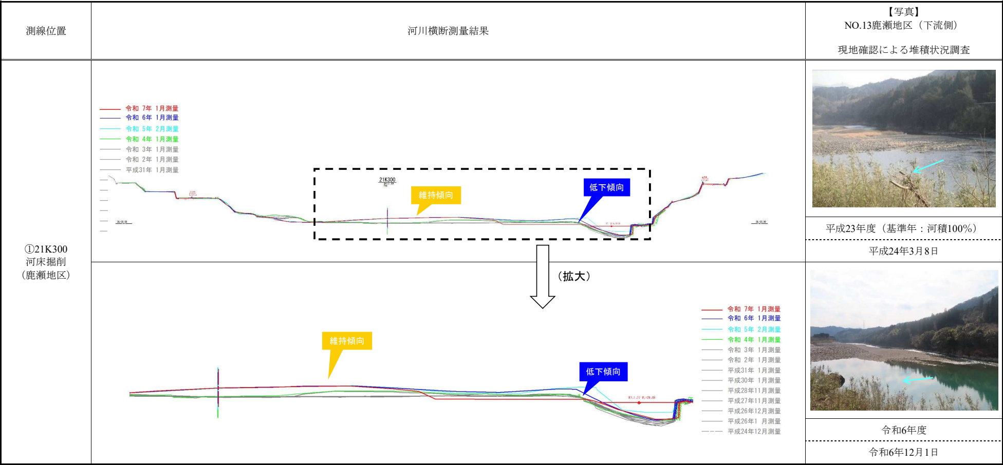
図 1-11 (1) 横断測量結果（治水安全度の評価対象箇所）
