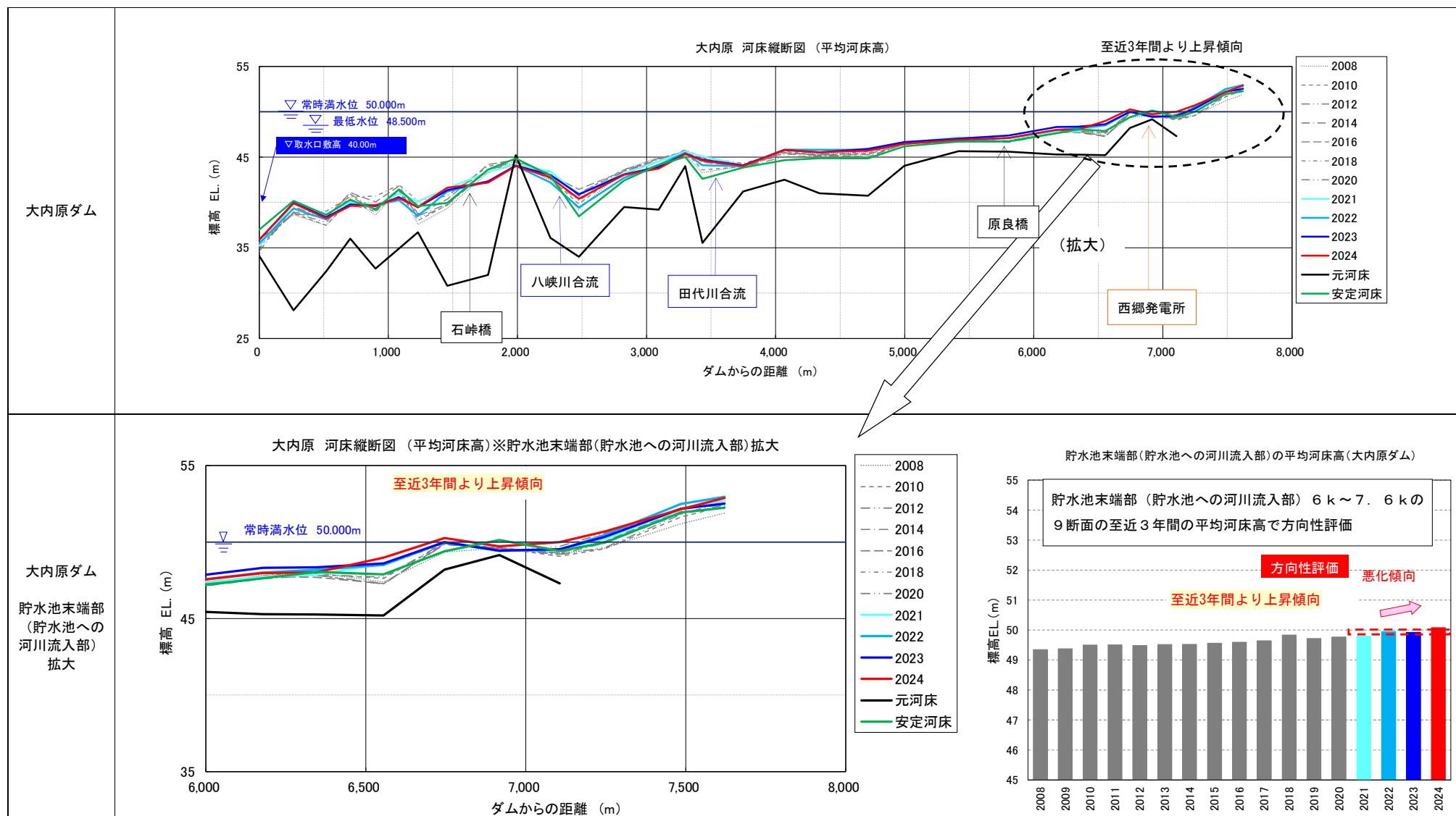
図9-9 ダム貯水池の堆砂形状（大内原ダム）
