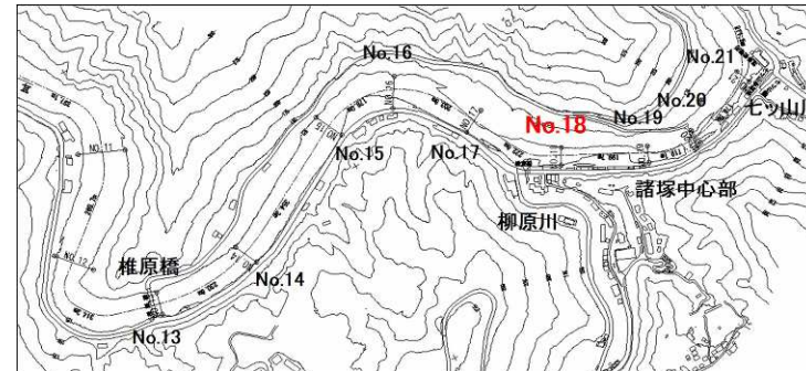
図9-6 検討断面位置図（No. 18）
