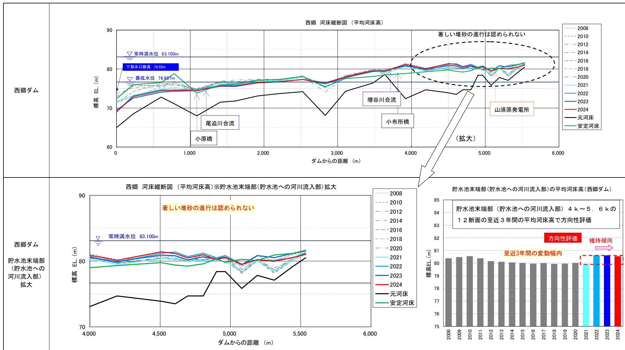
図9-8 ダム貯水池の堆砂形状（西郷ダム）
