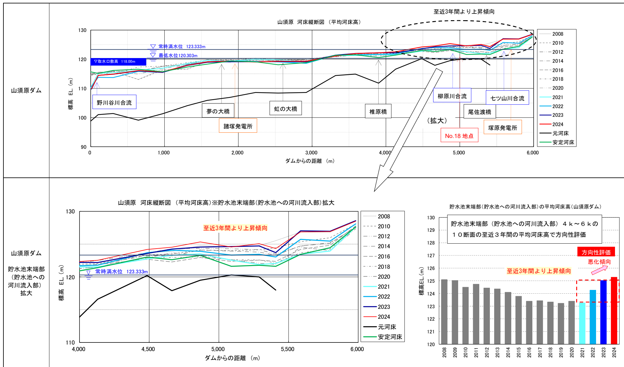
図9-5 ダム貯水池の堆砂形状（山須原ダム）
