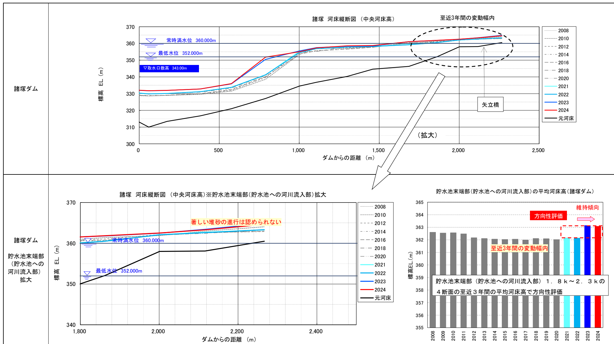
図9-10 ダム貯水池の堆砂形状（諸塚ダム）
