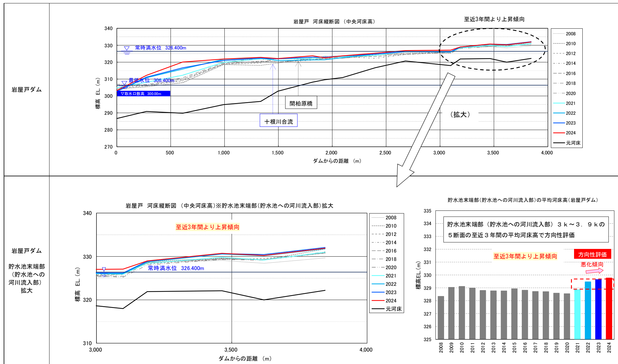
図9-3 ダム貯水池の堆砂形状（岩屋戸ダム）
