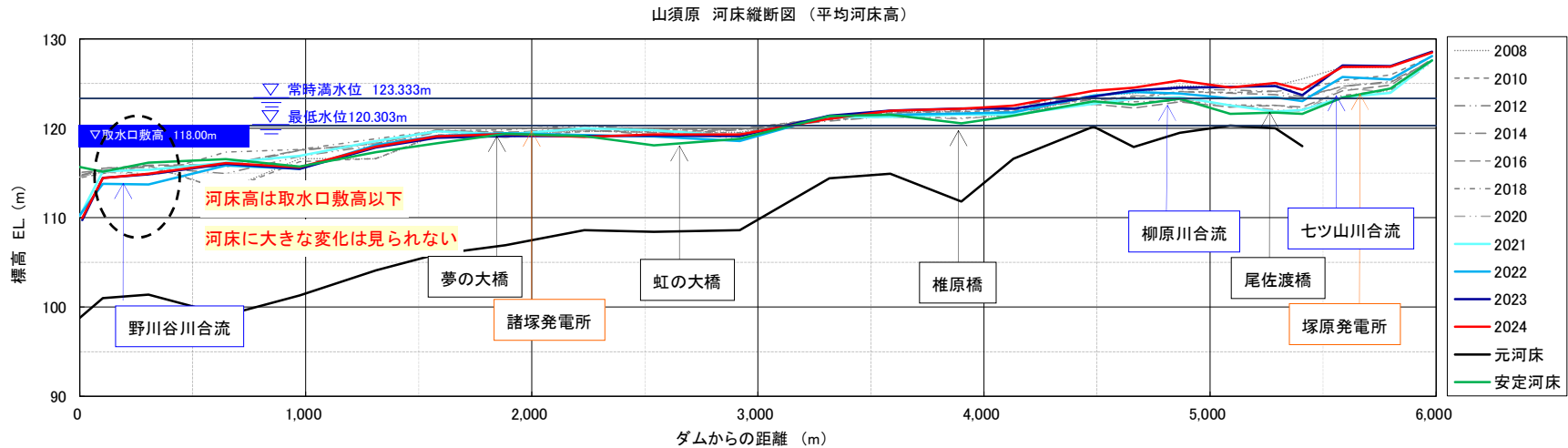
図11-2(2) ダム貯水池の堆砂形状（取水口の敷高と堆砂面の関係）
