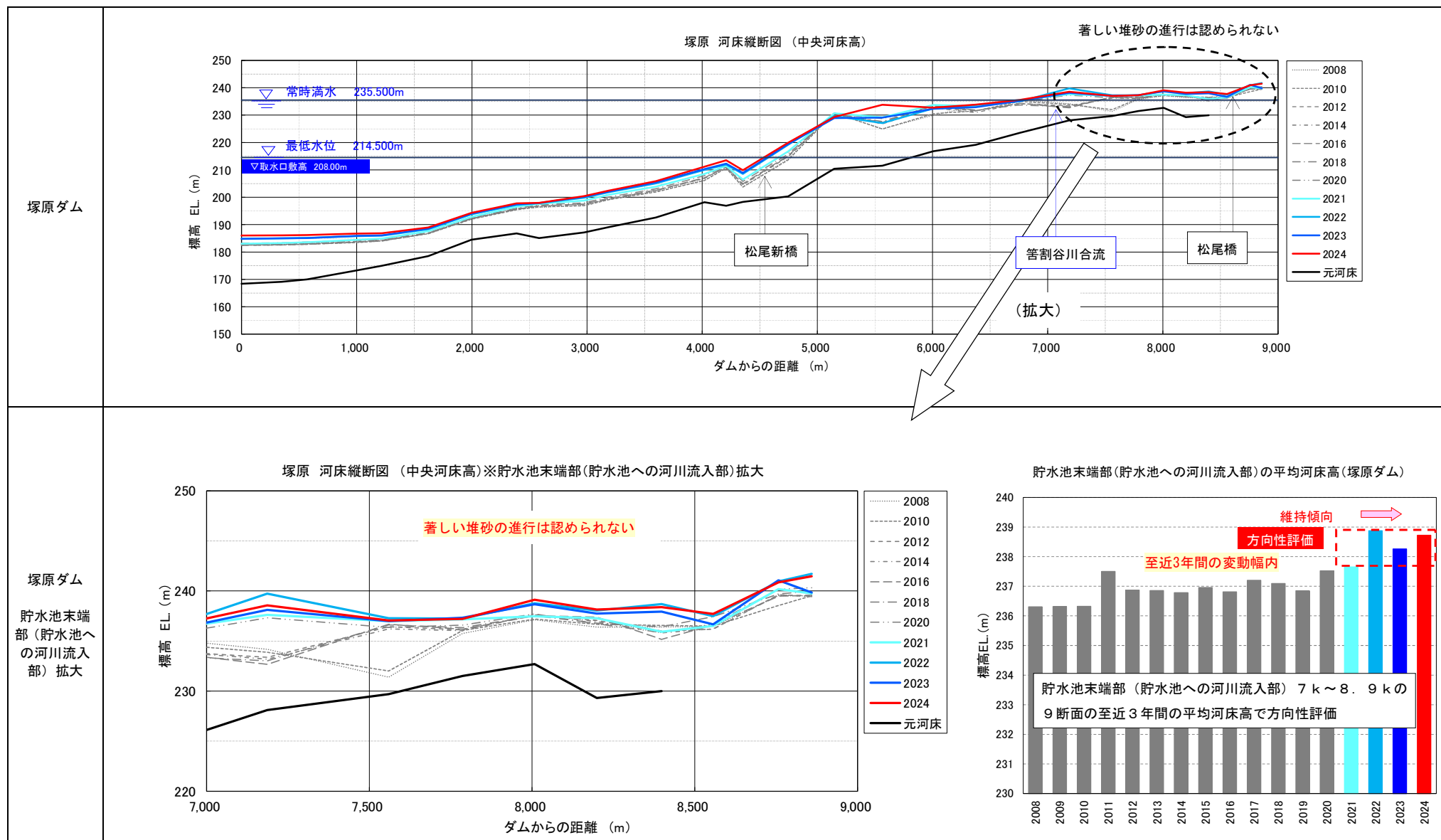
図9-4 ダム貯水池の堆砂形状（塚原ダム）
