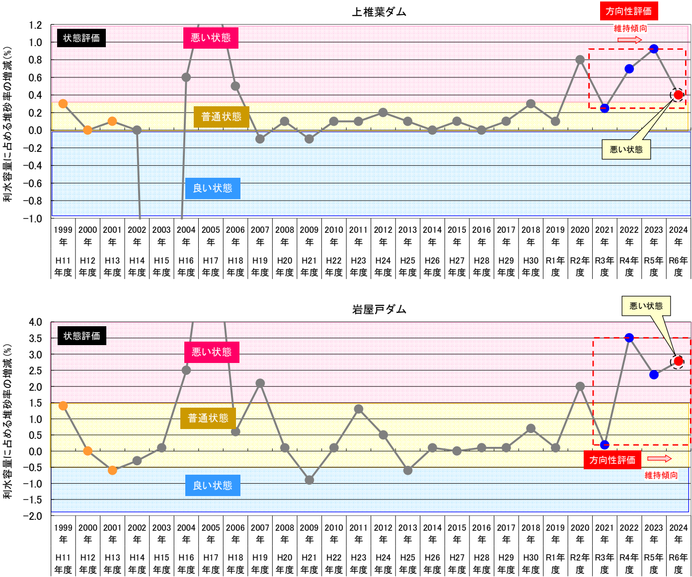
図10-2(1) 利水容量に占める堆砂率の増減の推移（上椎葉ダム、岩屋戸ダム）
