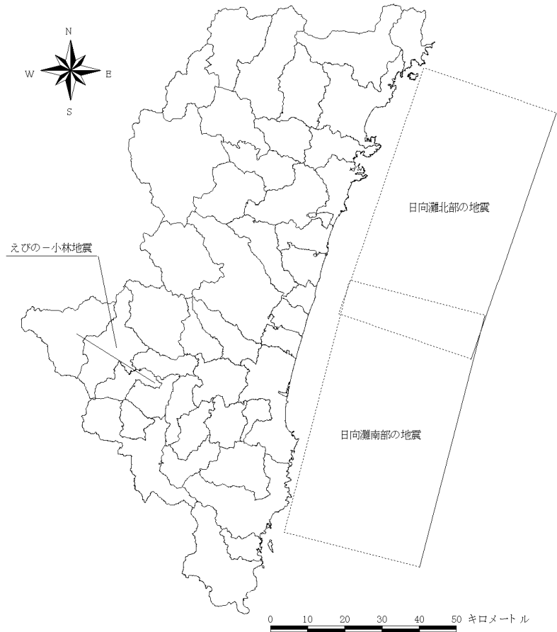
日向灘地震の発生確率
