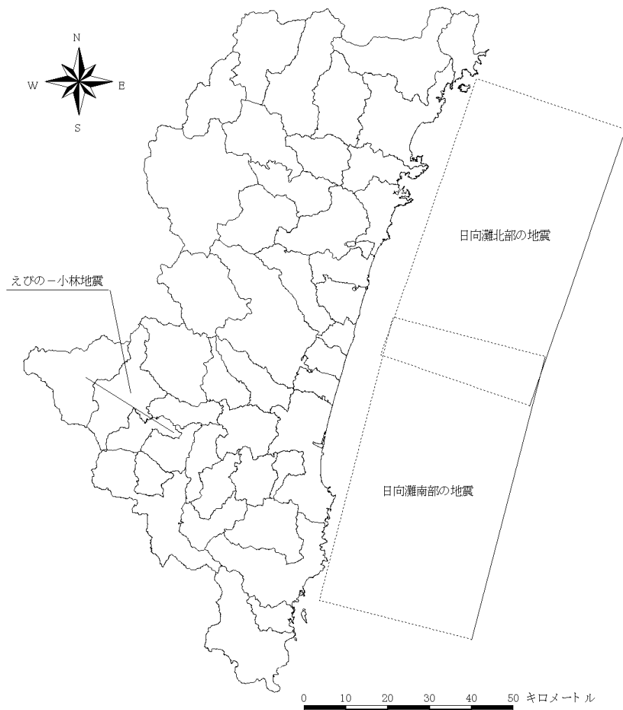
えびの・小林地震の想定震源域
