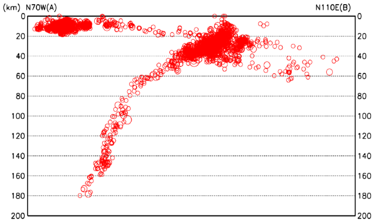
図 1-2 図 1-1 の破線 A—B からみた断面図
