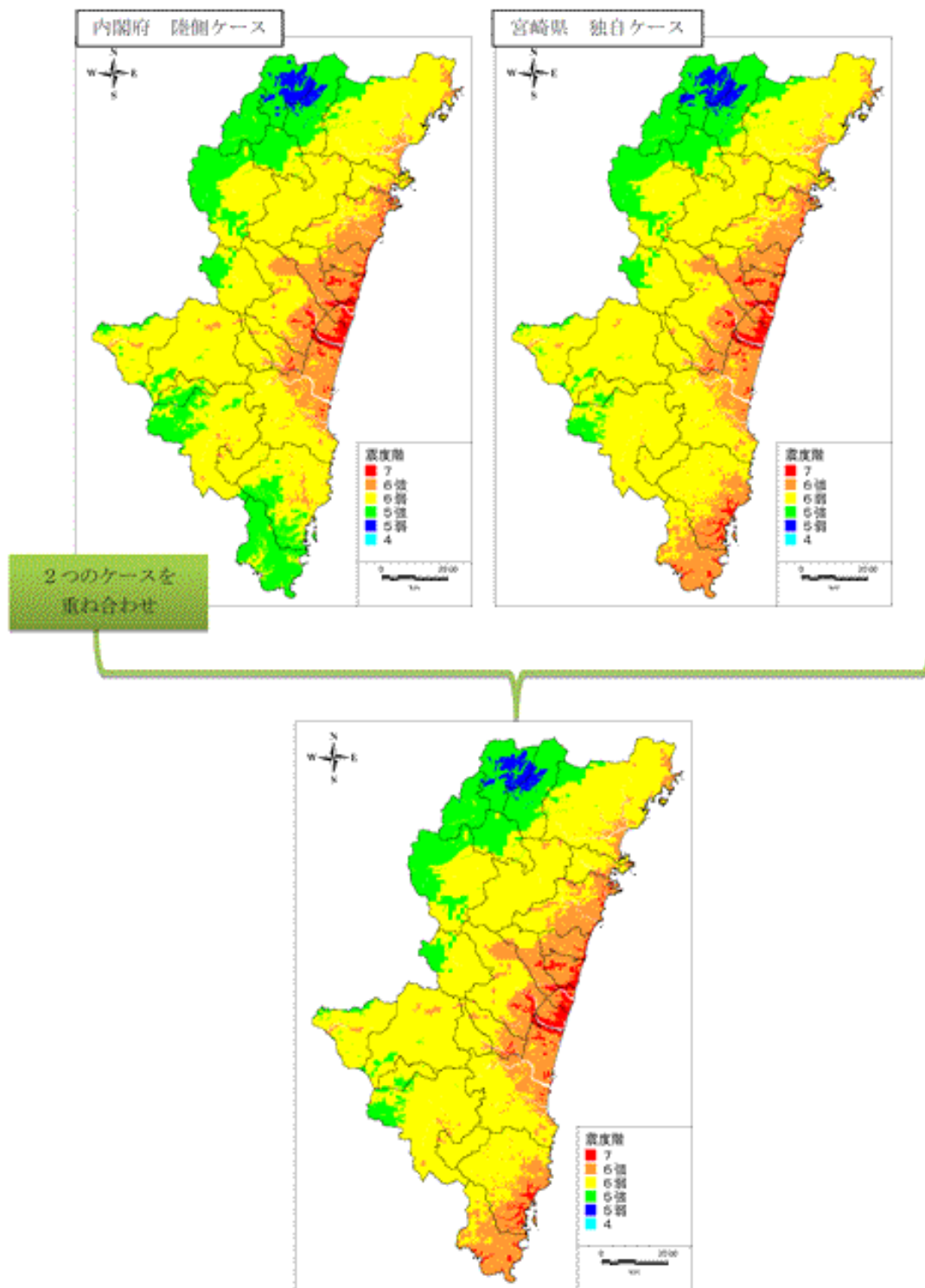
震度分布
