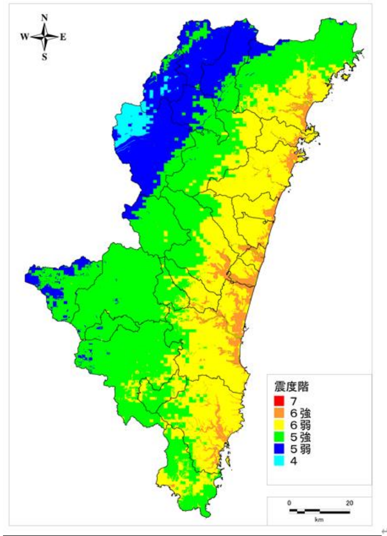
震度分布図（最大）
