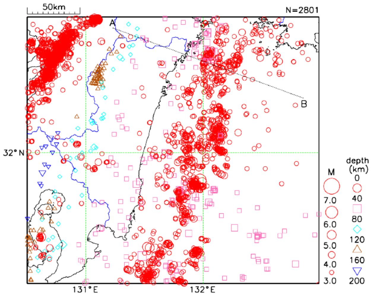
図 1-1 宮崎県周辺に発生した地震とその大きさ(1997.10.01~2023.12.31)
