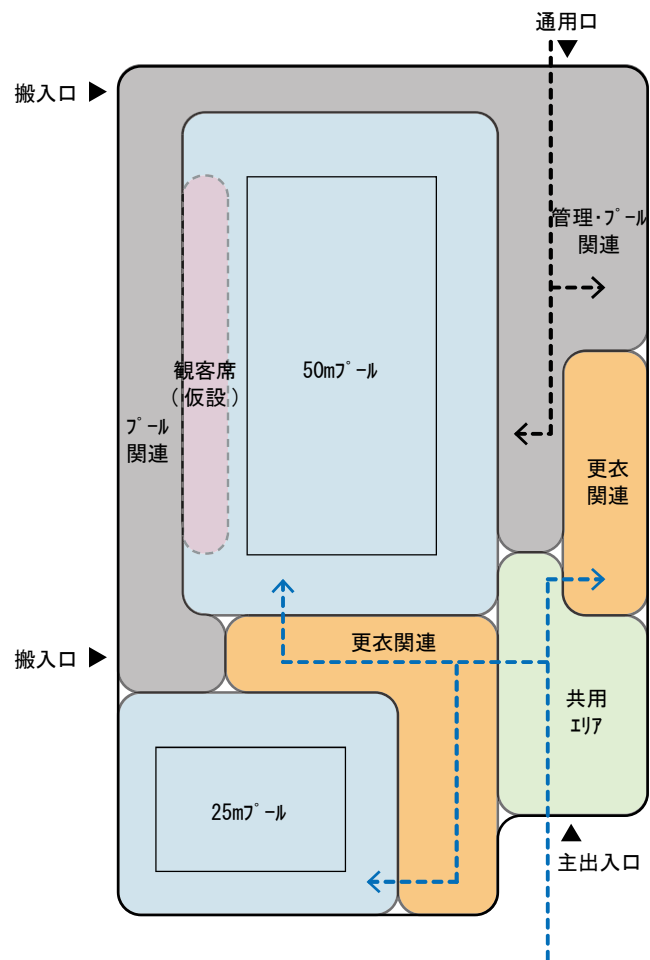
<1階平面>
