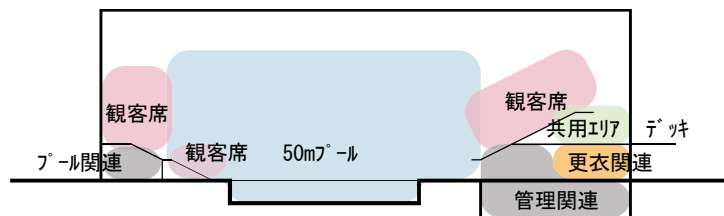
<断面>
