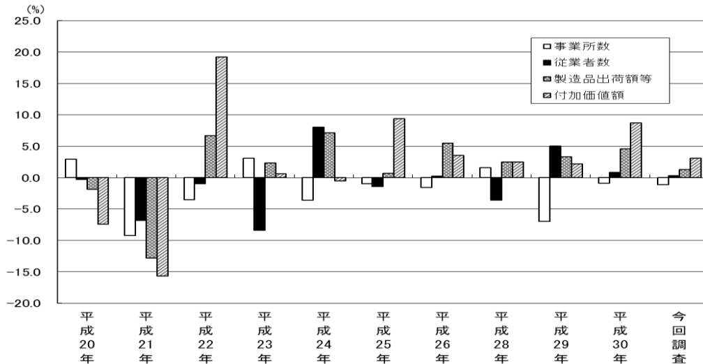
図 1-2 事業所数、従業者数、製造品出荷額等、付加価値額の推移における対前年増加率の推移 (従業者 4 人以上の事業所)
