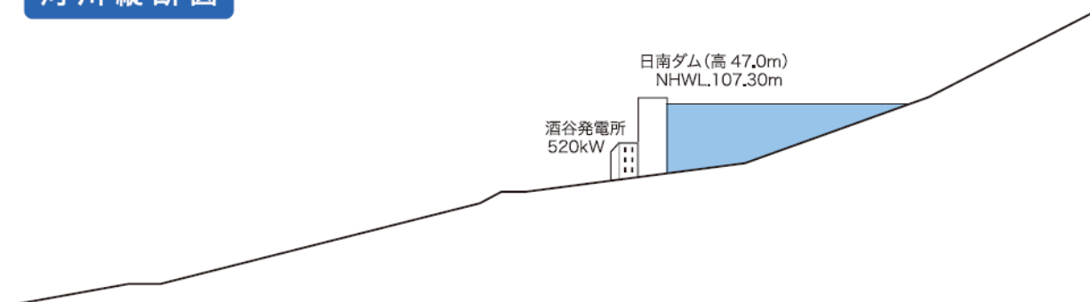
河川縦断図
