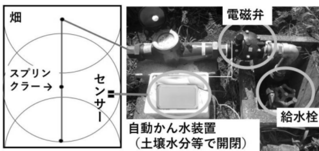
省力型自動かん水装置イメージ
