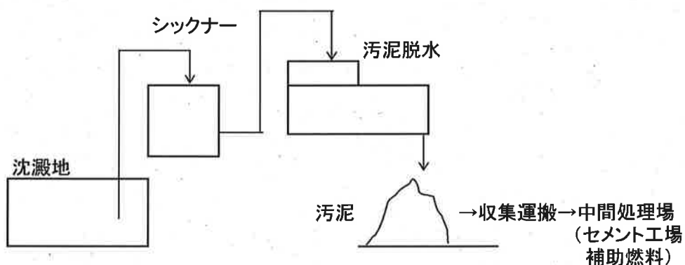
図 4 産業廃棄物の一連の処理の工程(汚泥)
