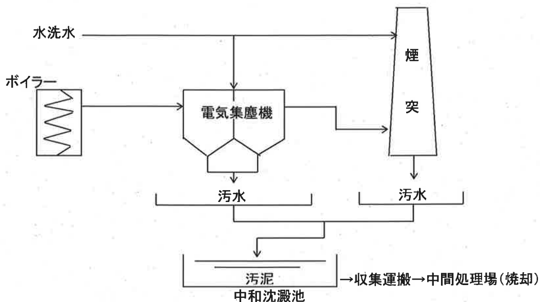
図 3 産業廃棄物の一連の処理の工程(汚泥)
