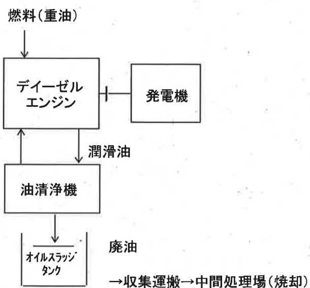
図 5 産業廃棄物の一連の処理の工程(廃油:ディーゼル発電機)
