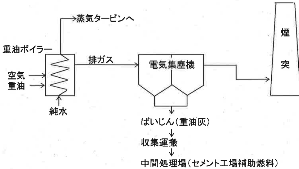
図 1 産業廃棄物の一連の処理の工程(ばいじん:重油灰)
