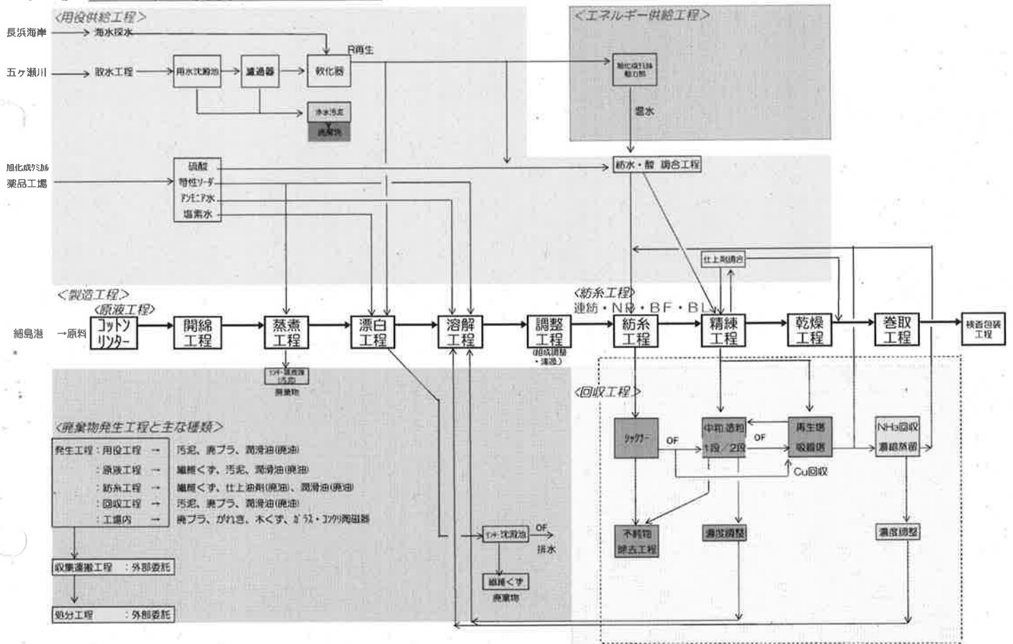
別図① ベンベルグ工場 廃棄物処理フローシート
