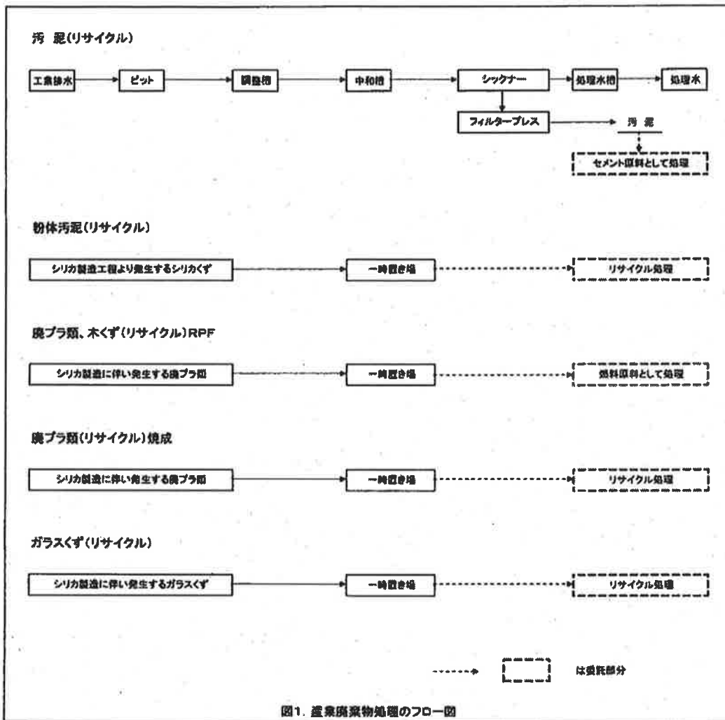
図1. 産業廃棄物処理のフロー図
