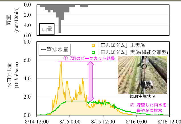
水田からの流出量抑制効果（実証事業 観測結果）
