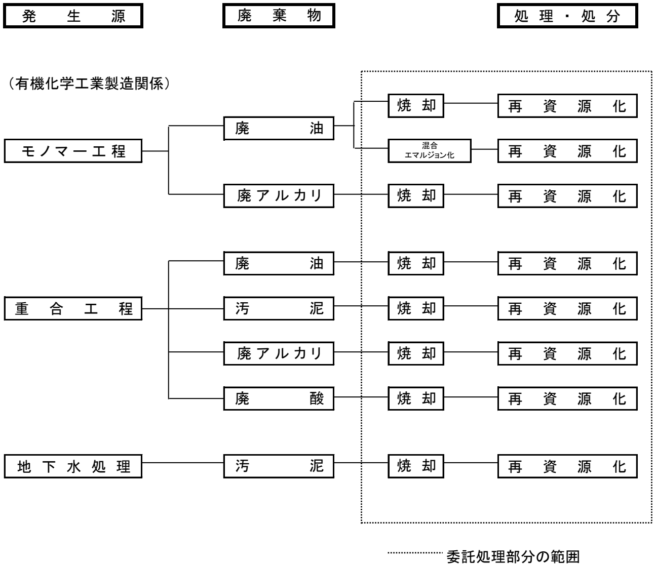
特別管理産業廃棄物処理フロー図
