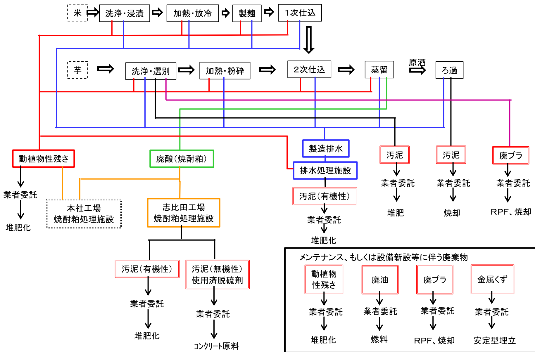
別添 図1 産業廃棄物の一連の処理工程(志比田、志比田増設、志比田第二増設工場:焼酎製造)
