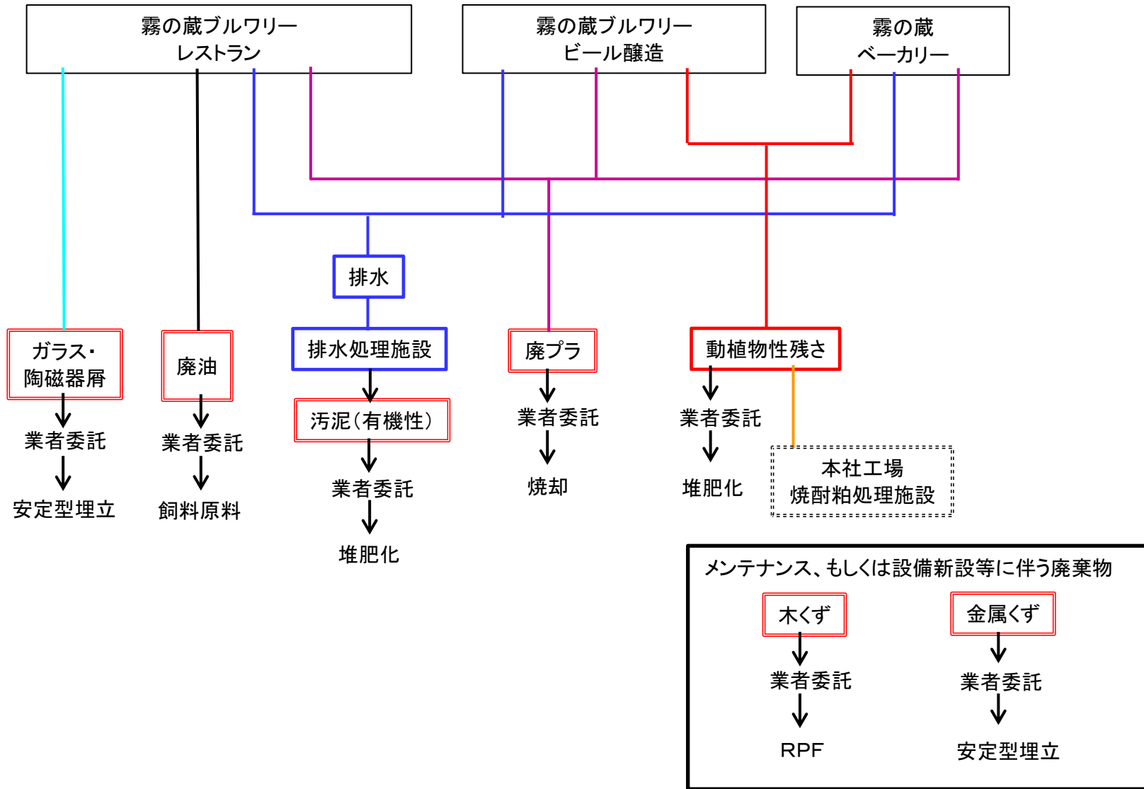
別添 図2 産業廃棄物の一連の処理工程(志比田工場 霧の蔵ファクトリーガーデン)
