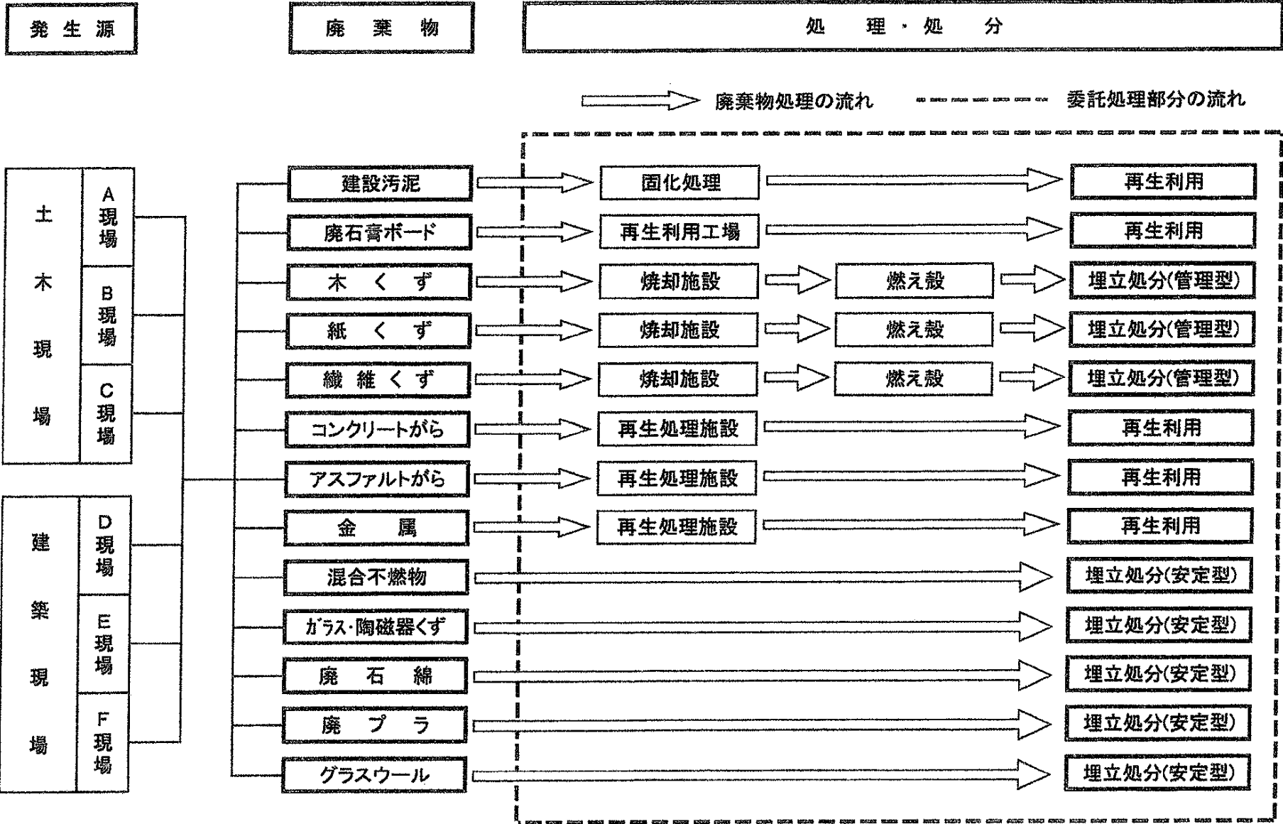
廃棄物処理フロー図(現状)
