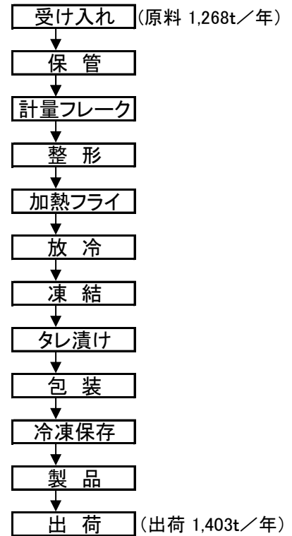
図4 惣菜工場フローシート (惣菜工場)
