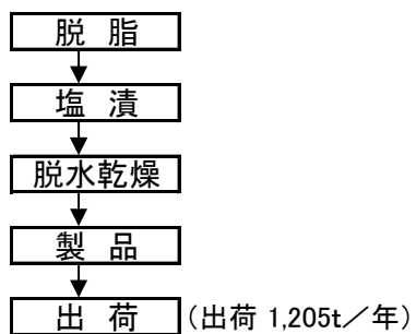
図5 原皮工程フローシート (原皮工場)
