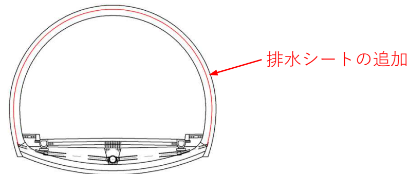
湧水処理対策 (排水シート)
