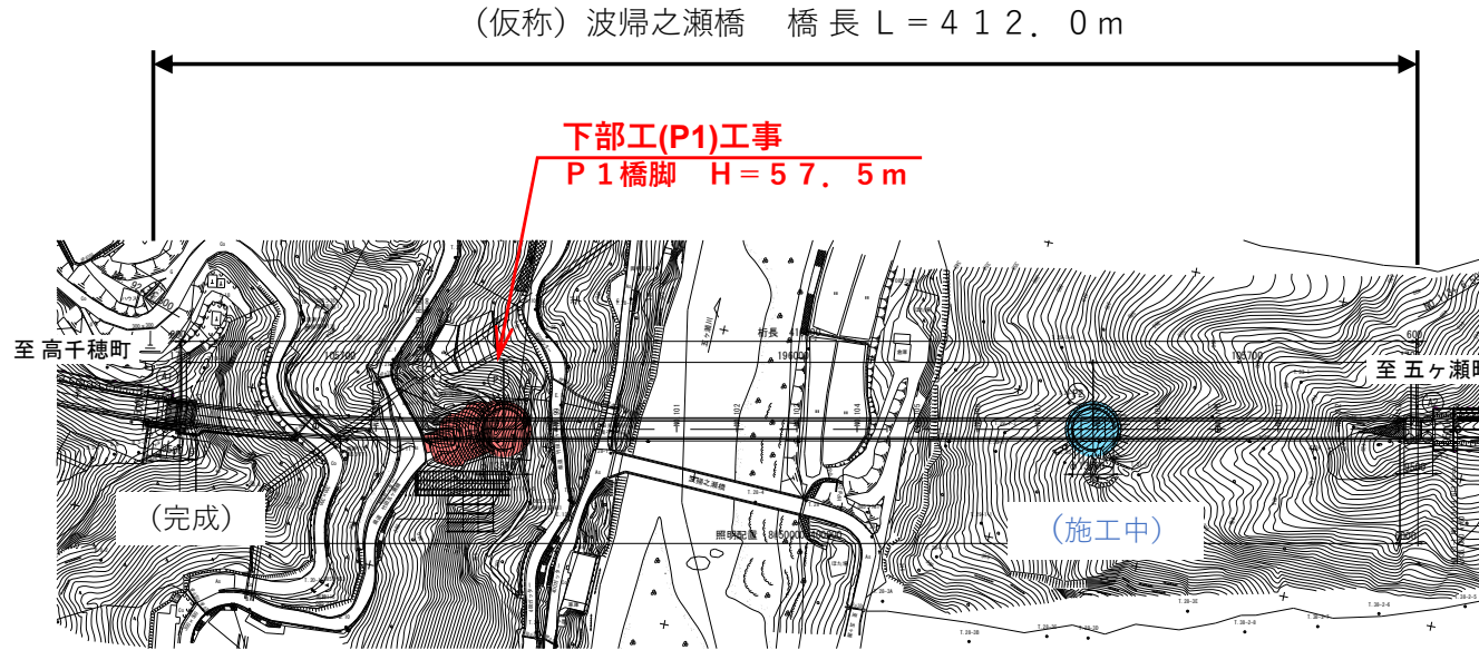
平面図
