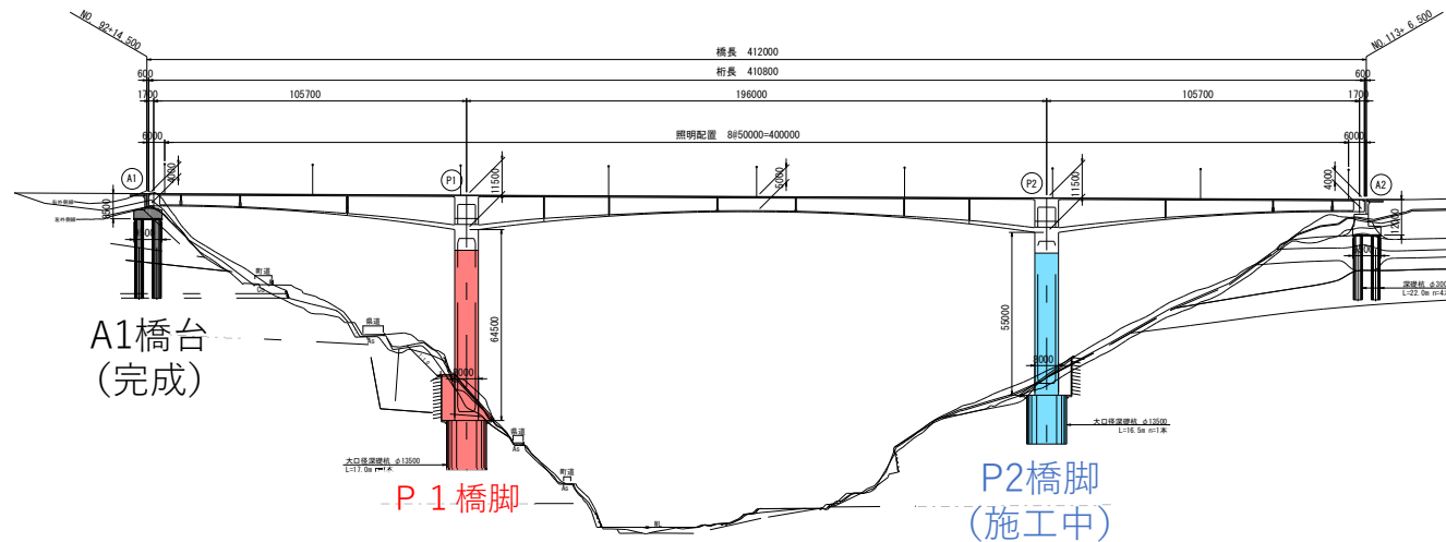
側面図
