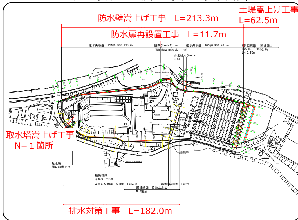
中野原浄水場浸水対策工事平面図
