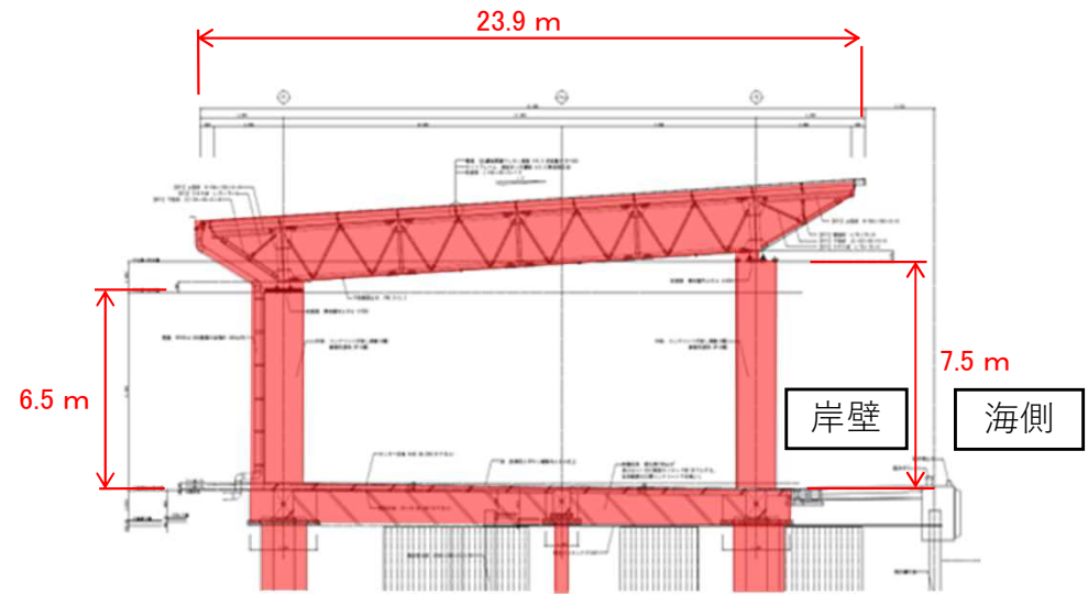
断面図
