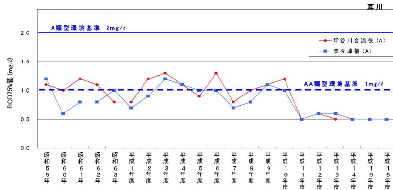
図-2 主要地点における水質(BOD75%値)の経年変化
