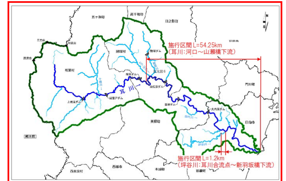
図-5 施行区間（全体図）
