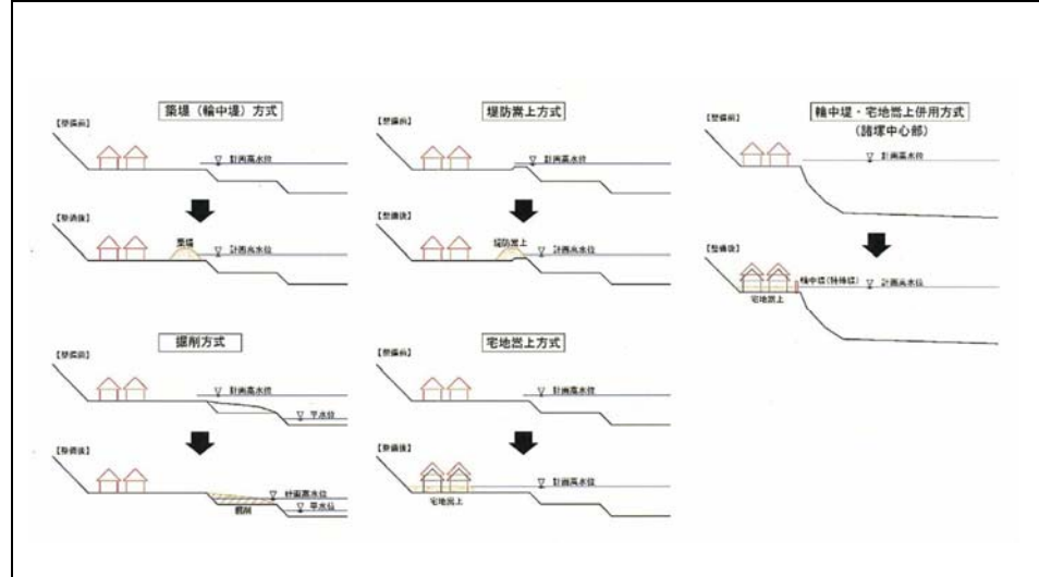
図-7 工法別模式
