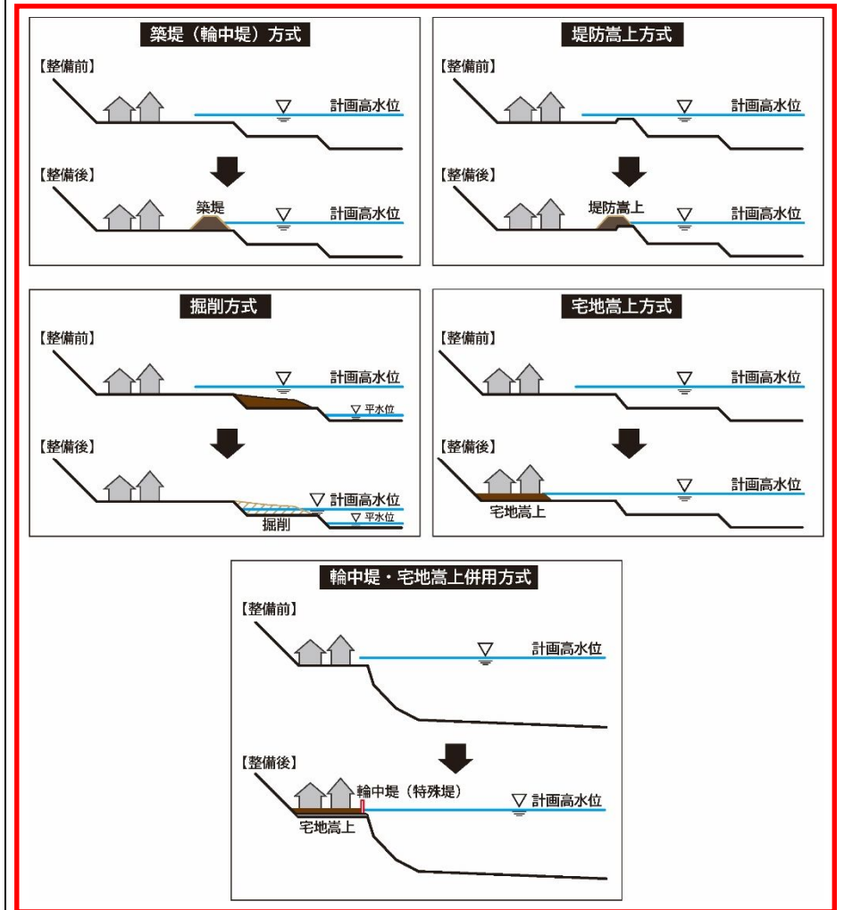
図-9 治水対策方式イメージ図
