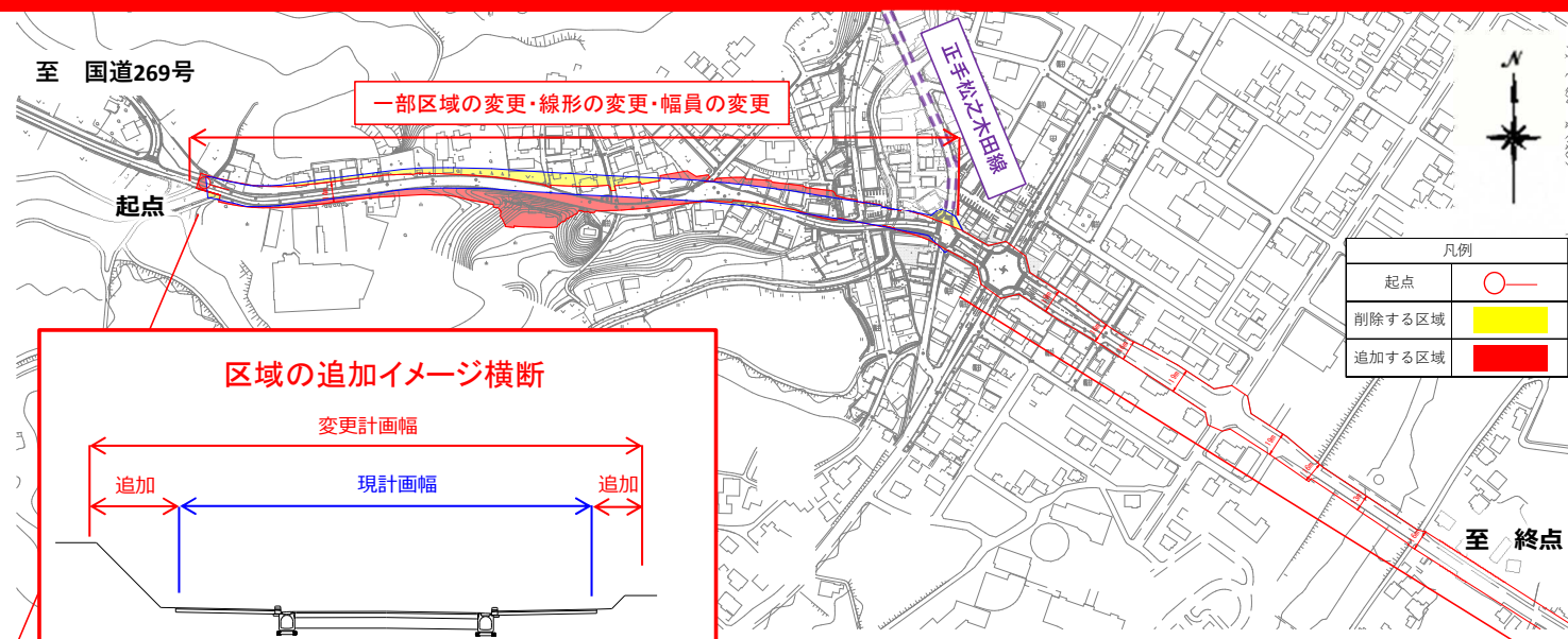
一部区域の変更（拡大図）
