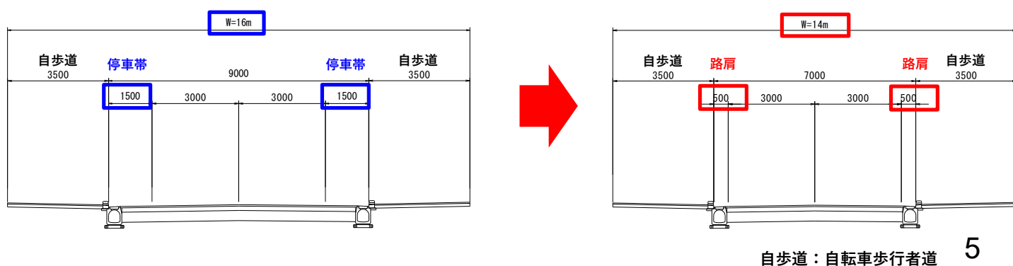
都市計画横断図
