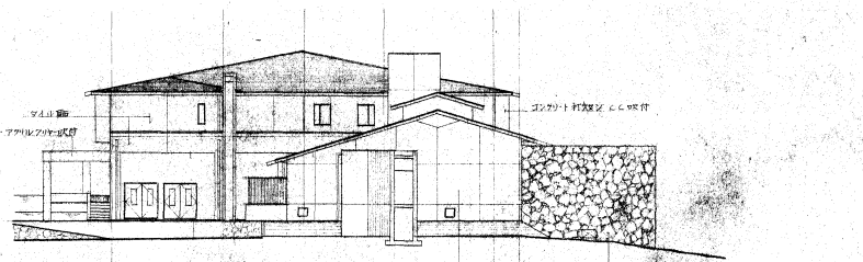
西面図
