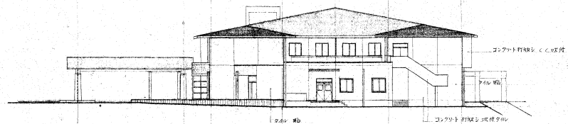
東面図
