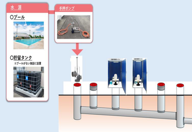
マンホールトイレ ～イメージ～
