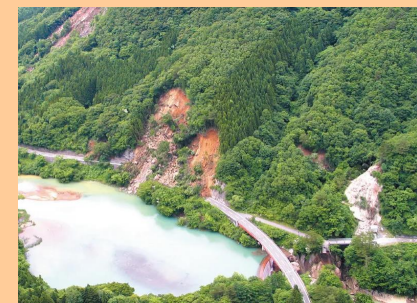
土砂災害
